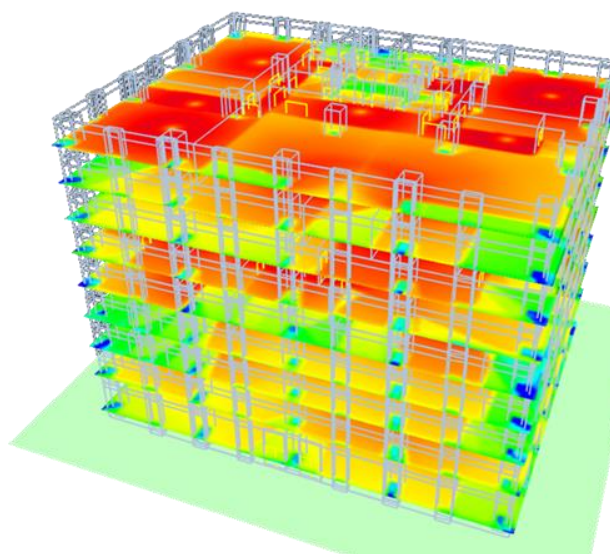
'Heat map' som visar prognosticerad täckning av ett 4G(LTE) trådlöst nätverk inomhus.
